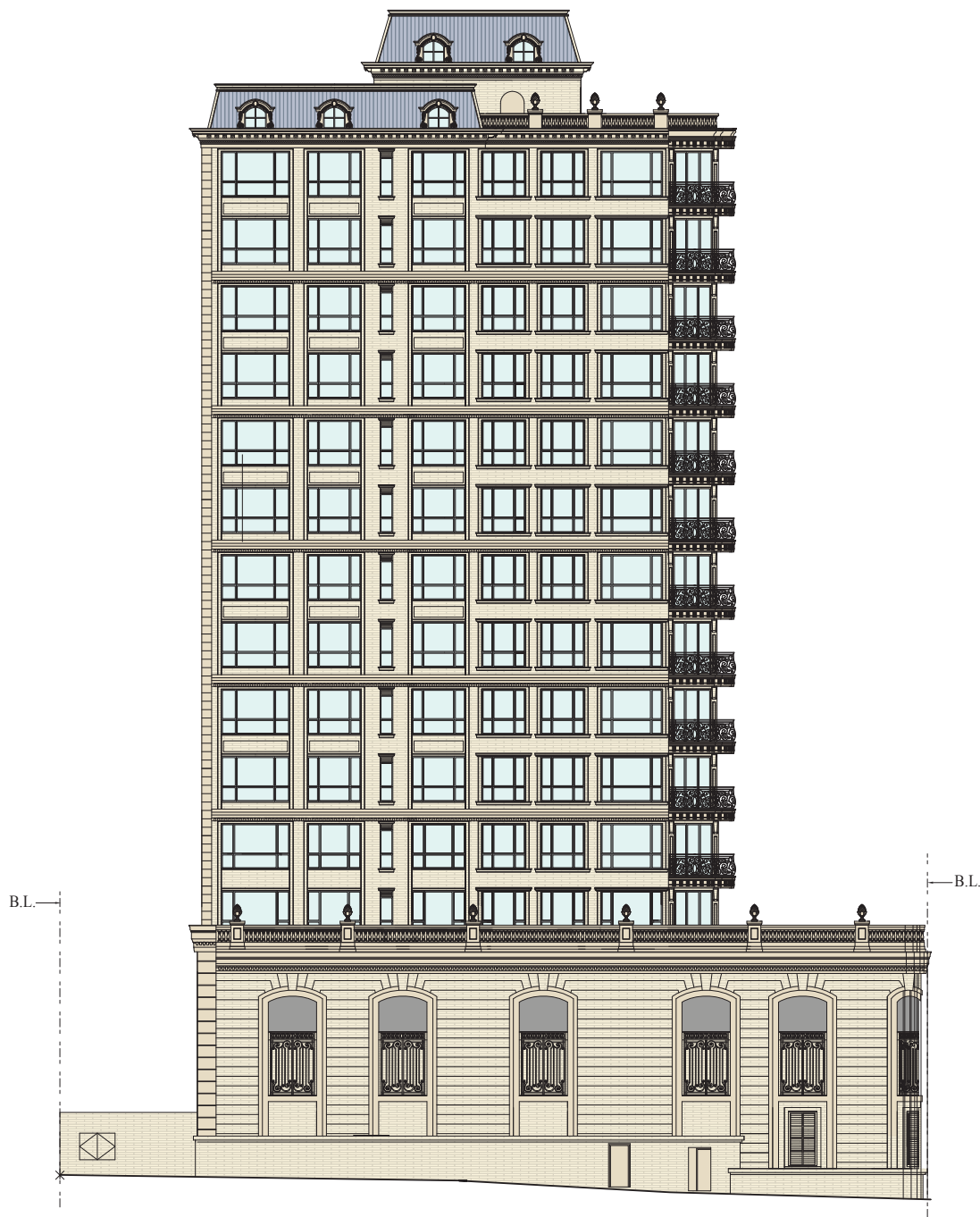
東南面立面圖 SOUTH EAST ELEVATON
